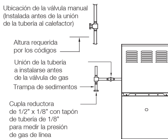
Fig. 24 - Arreglo típico de la tubería de gas
