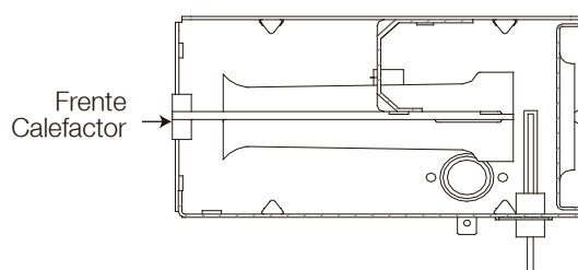
Fig. 33 - Posición del encendedor - 2
