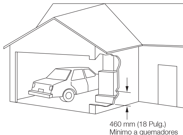
Fig. 4 - Instalación en garaje
