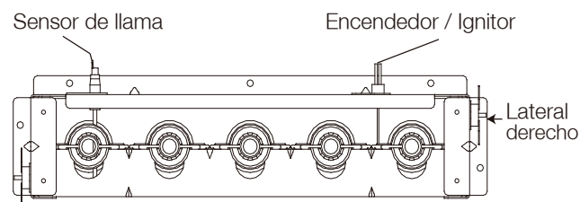
Fig. 32 - Posición del encendedor - 1
