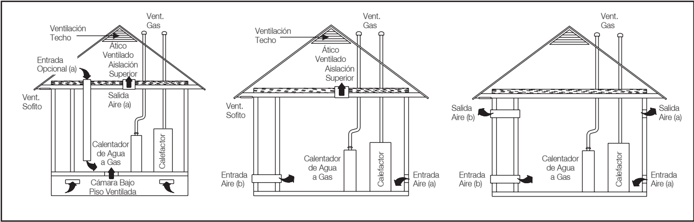
Fig. 22 - Aire de combustión exterior y del ambiente
