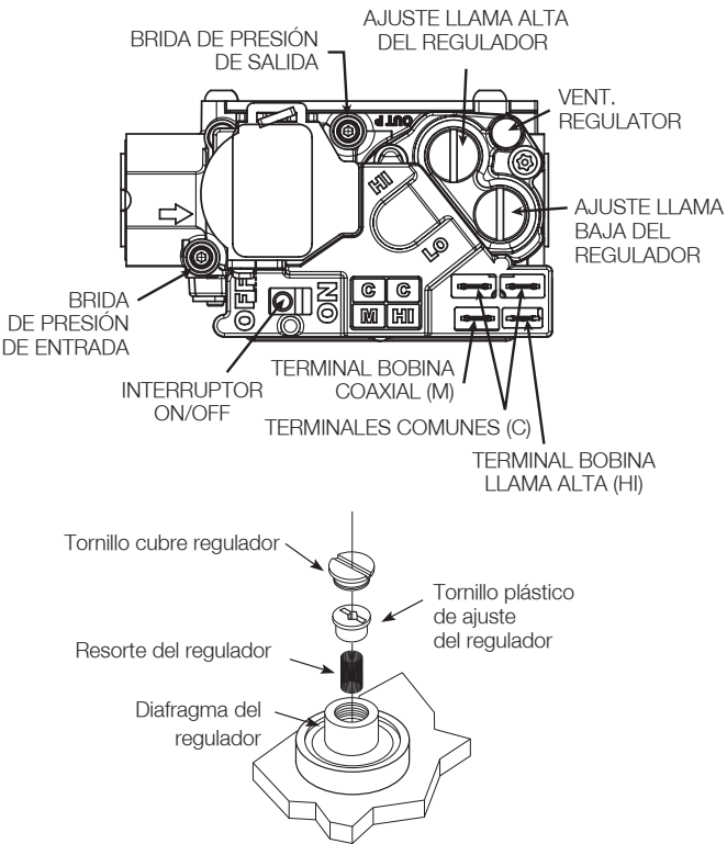
Fig. 28 - Ajuste de la válvula y el regulador de gas
