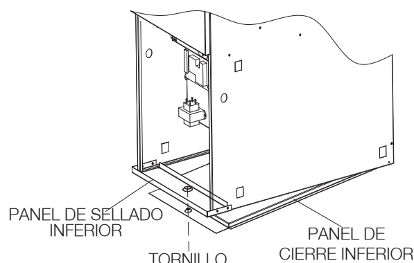
Fig. 5 - Extracción del panel de cierre inferior
