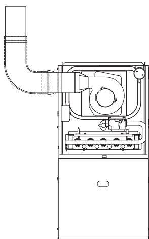
Fig. 16 - Aplicación de flujo ascendente Codo de ventilación izquierdo
